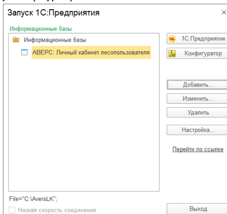
Рисунок 9. Запуск Конфигуратора.
