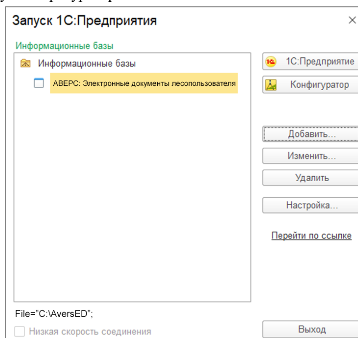
Рисунок 9. Запуск Конфигуратора.
