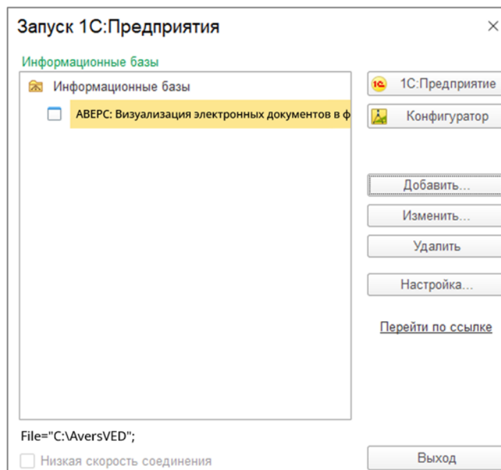
Рисунок 9. Запуск Конфигуратора.
